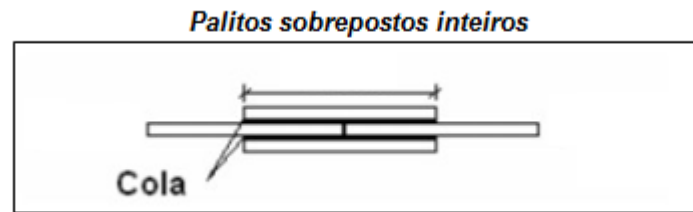
Figura 1 – Esquema de emenda das barras
